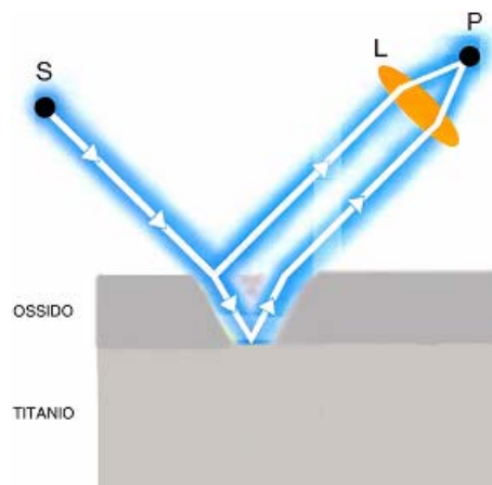
Figura 1 – Fenomeni di interferenza ottica su titanio anodizzato
